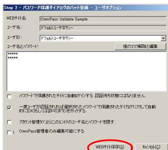
Fig. 4-21 サーバー側管理コンソール
