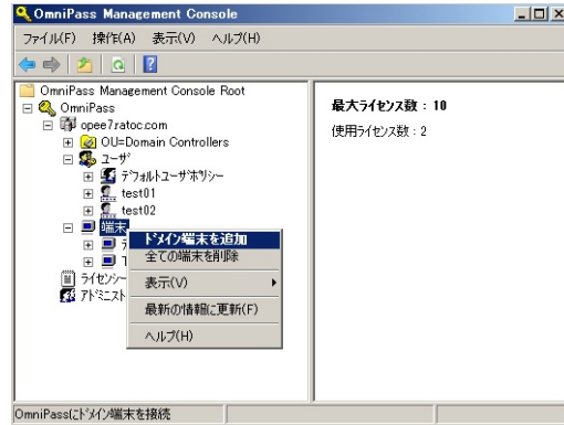
OmniPassEE 管理コンソールから登録
