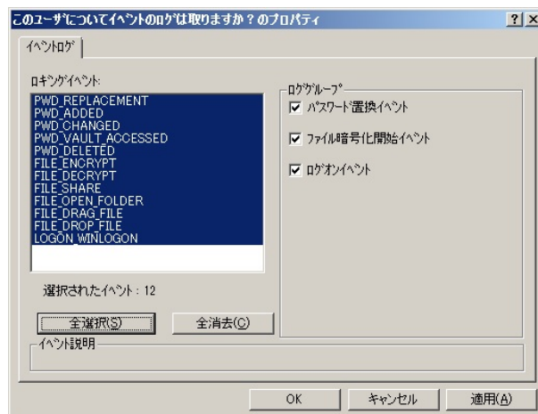
Fig. 3-73 サーバー側管理コンソール
