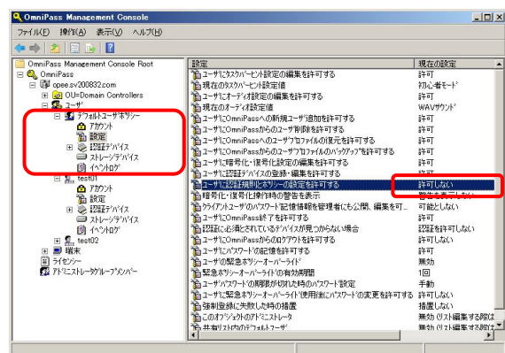
Fig. 4-43 サーバー側管理コンソール
